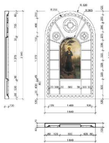
Рисунок 6. Проект киота
