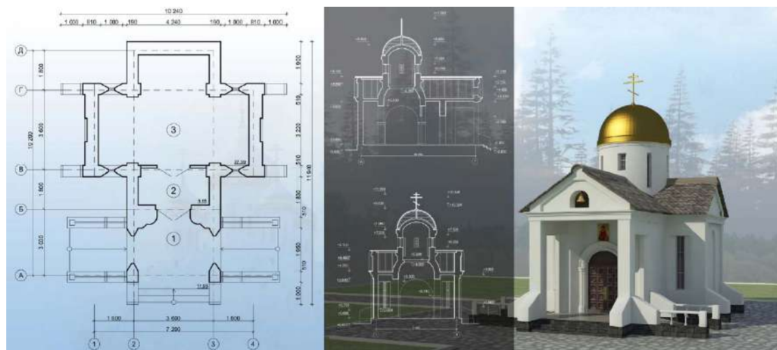
Рисунок 2. Архитектурно-планировочное решение проектируемого объекта
