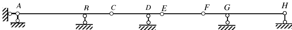
Рис. 13. Многопролетная балка
