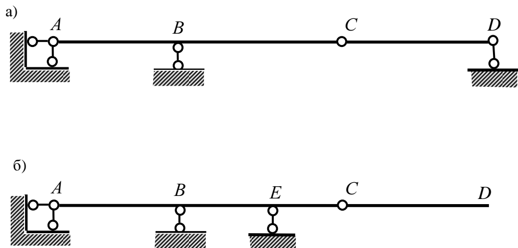
Рис. 6. Шарнирно консольные системы
