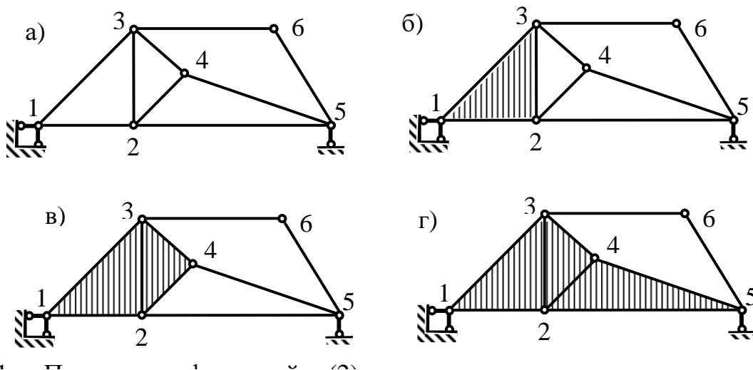
Рис.10. Последовательность анализа структуры шарнирно стержневой системы V = 6 , C = 9 , C_o = 3 , W = 2 \cdot 6 - 9 - 3 = 0 , следовательно, система имеет
