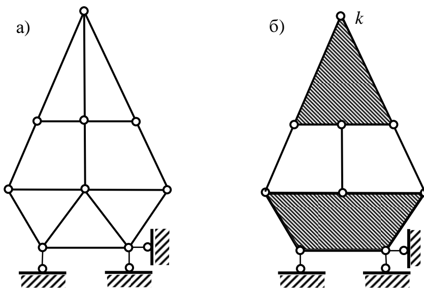
Рис. 12. Шарнирно-стержневая система
