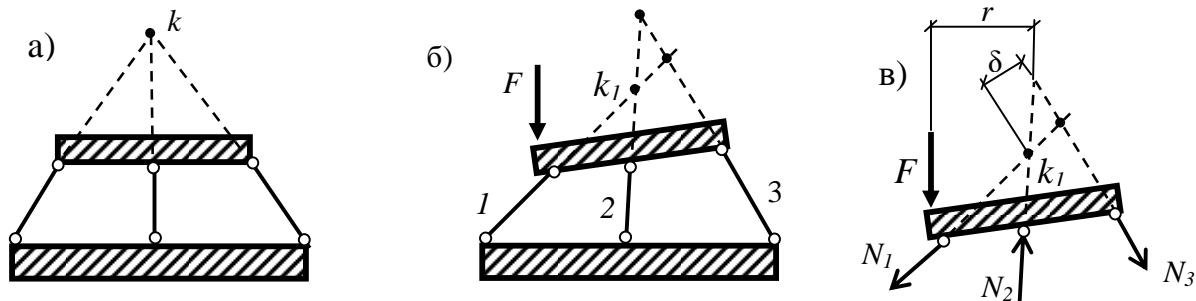
Рис.8. Определение усилий в системе, близкой к мгновенно изменяемой
