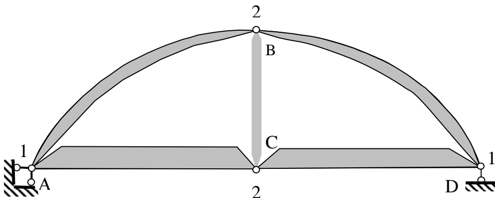
Рис. 11. Система с кратными шарнирами
