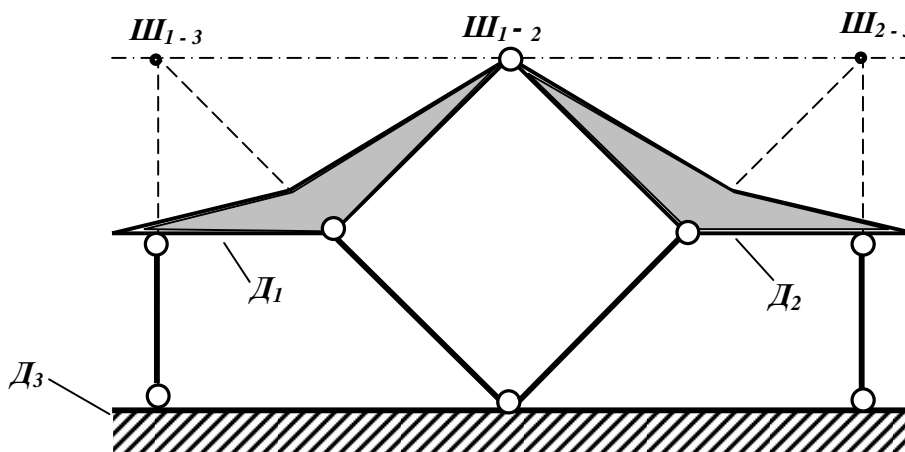
Рис. 14. Мгновенно изменяемая система
