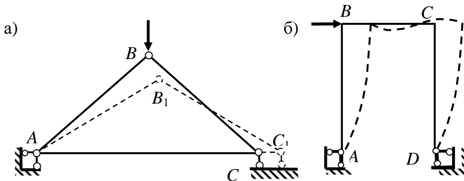
Рис. 1. Изменение формы систем, вызванное деформацией элементов
