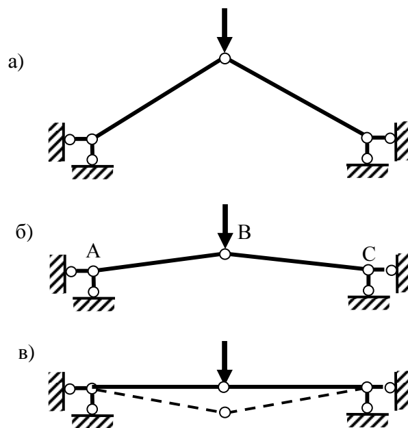
Рис.7. Превращение системы в мгновенно изменяемую
